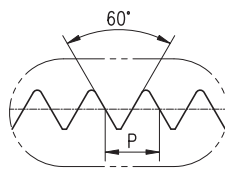
Detalhe do perfil da rosca
